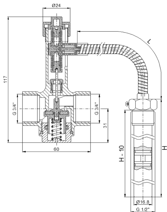
ROZMĚROVÉ SCHÉMA
